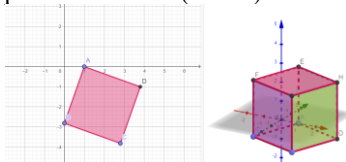
Рис.1 Приклад 3D моделі, побудованої за допомогою GeoGebra
