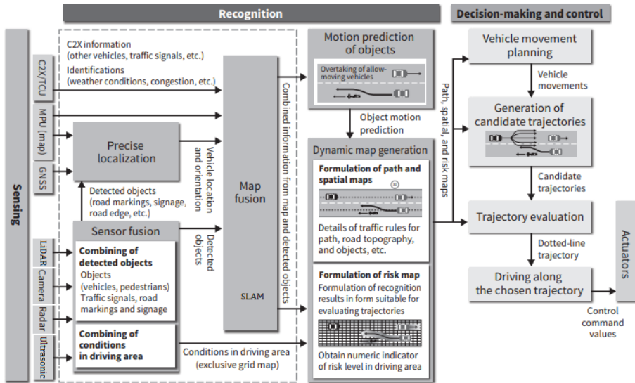
Рис. 9 Блок-схема системи навігації SDC.
