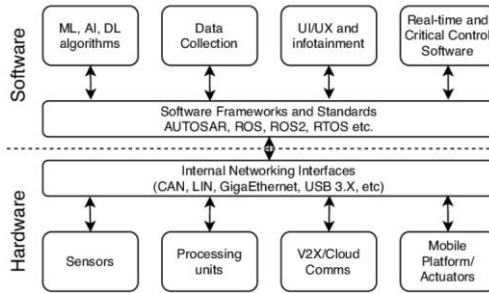
Рис. 6 Технічна архітектура системи навігації SDC.
